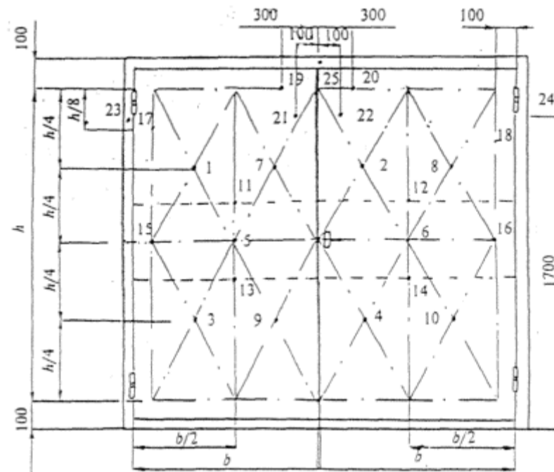
Рисунок 1 - Схема установки термоэлектрических преобразователей (термопар) на необогреваемой поверхности однопольных дверей
