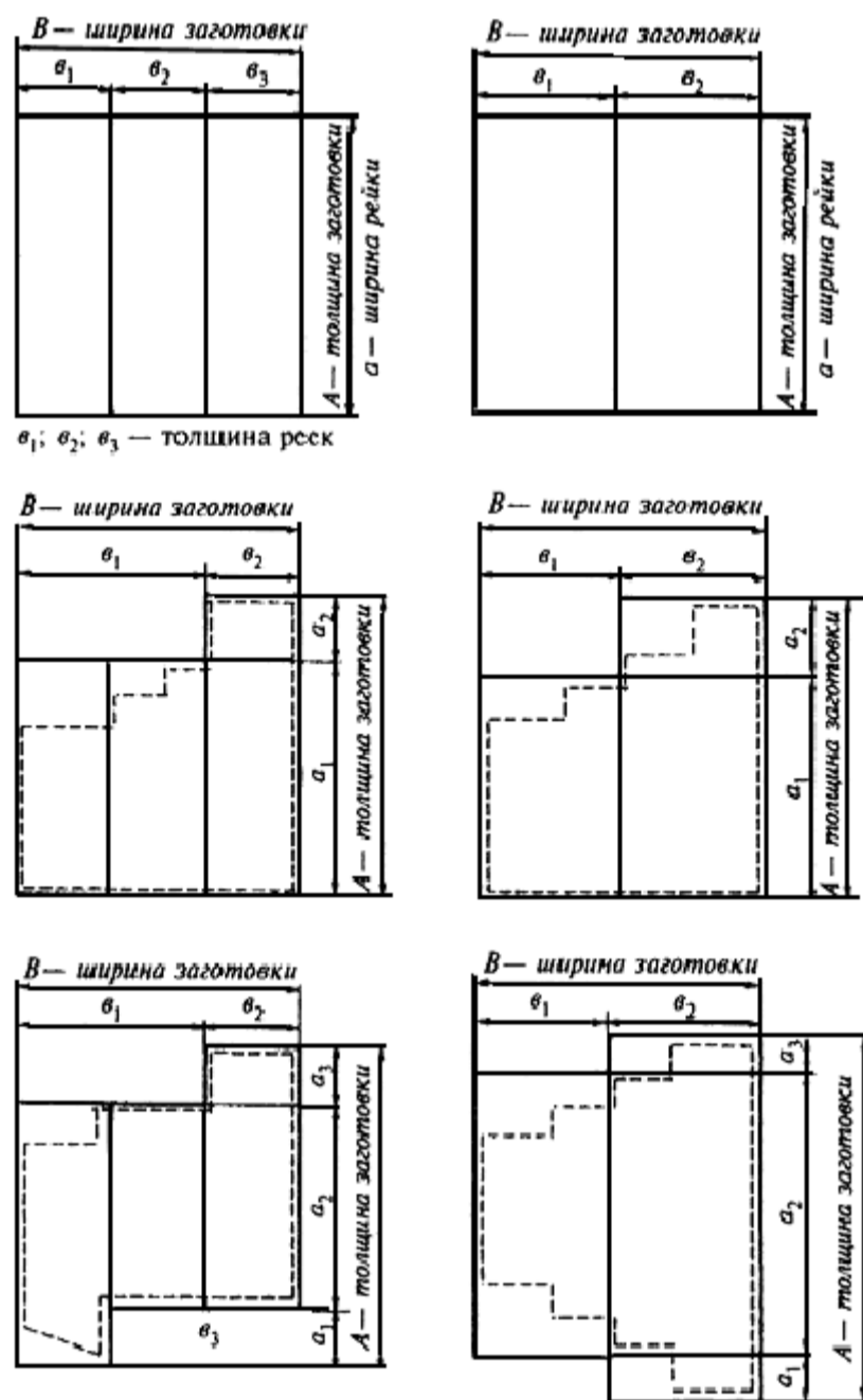
A; B; a^1; a^2; a^3; v^1; v^2; v^3 - контролируемые размеры
