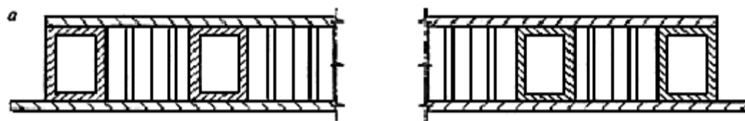
Полотно с двумя стальными листами, стальными профилями коробчатого сечения и сотовым заполнением
