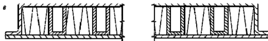
Полотно с наружным стальным листом и внутренним листом из ДВП, с профилями сложного сечения и заполнением из древесного или минерального утеплителя
