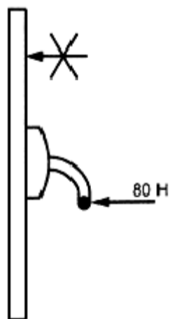
Рисунок В.5 - Схема приложения усилия для вывода засова из запорной планки устройства "Антипаника"
