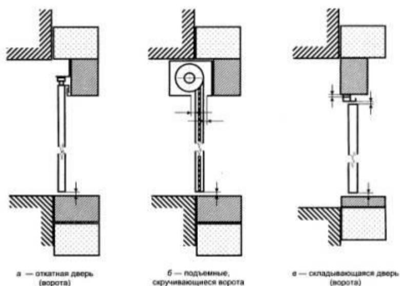
Рисунок 27 - Примеры замеров зазоров (вертикальное сечение)
