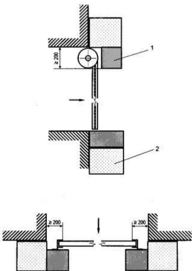
Рисунок 8 - Схема монтажа образцов складывающейся двери
