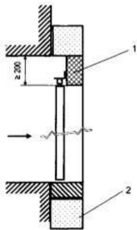
Рисунок 6 - Схемы монтажа образцов распашных дверей (вертикальное сечение)
