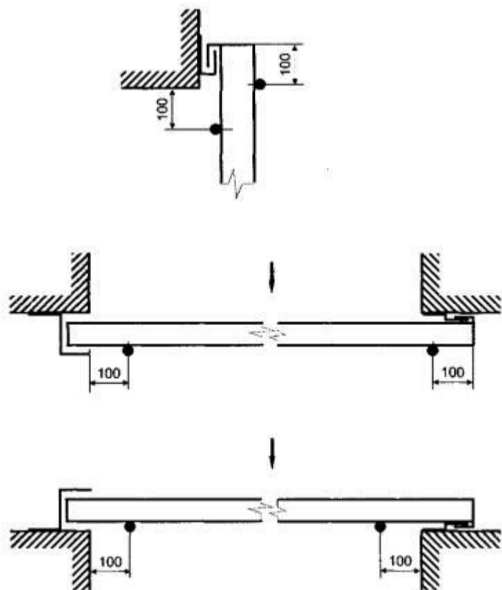
Рисунок 14 - Схема установки термодатчиков на необогреваемой поверхности полотна откатной двери (ворот)
