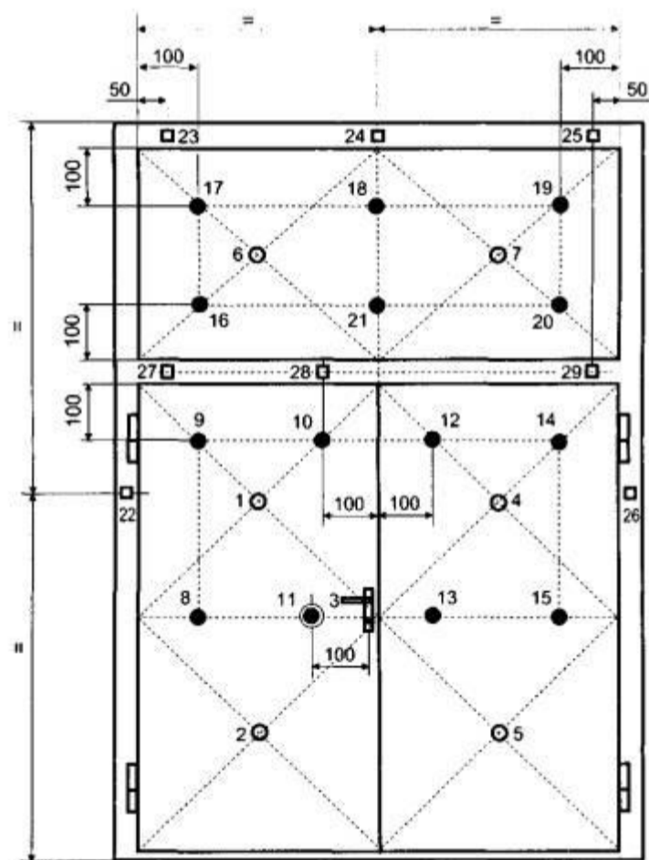
Рисунок 19 - Схема установки термодатчиков на неотапливаемой поверхности распашной двупольной двери с симметричными полотнами по ширине и с фрамгой
