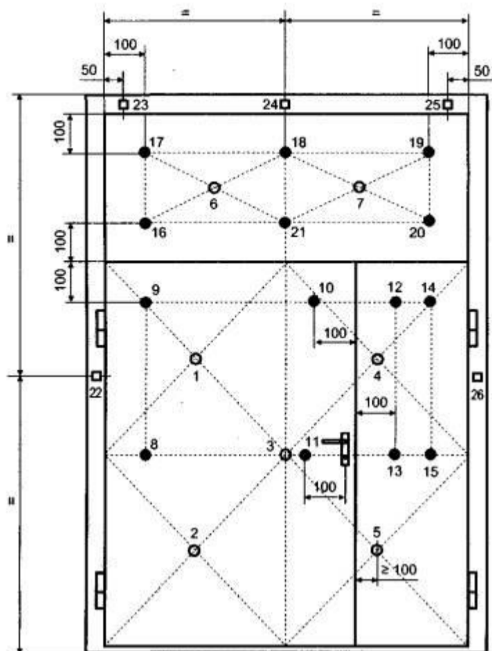
Рисунок 18 - Схема установки термодатчиков на неотапливаемой поверхности распашной двупольной двери (ширина полотен различная) с фрамгой
