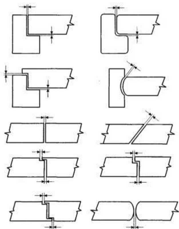
Рисунок 25 - Примеры замеров зазоров распашных дверей (горизонтальное сечение)
