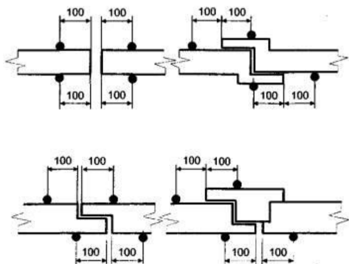
Рисунок 12 - Схема установки термодпар на необогреваемой поверхности полотна распашной однопольной двери в зоне 100 мм от его торцевых поверхностей и проема в свету (горизонтальное сечение)
