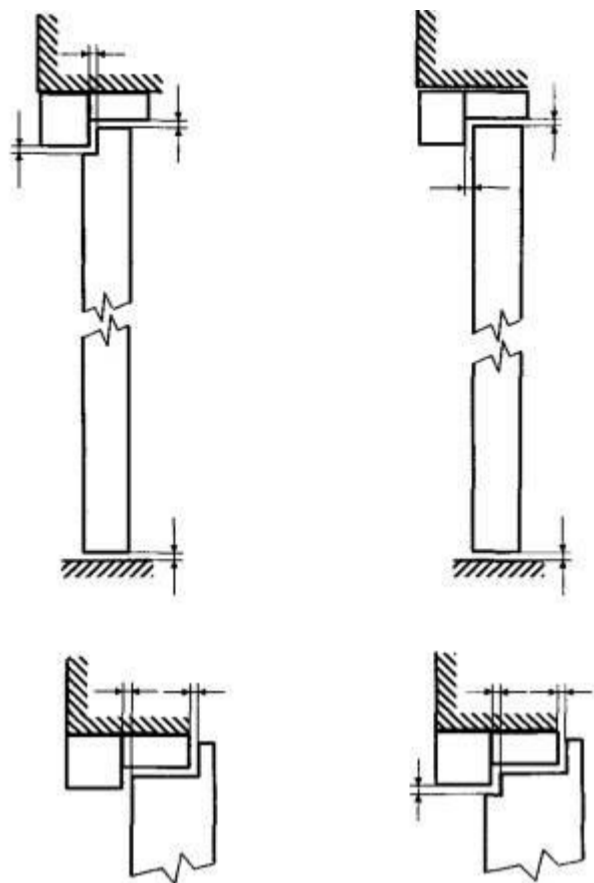
Рисунок 24 - Примеры замеров зазоров распашных дверей (вертикальное сечение)
