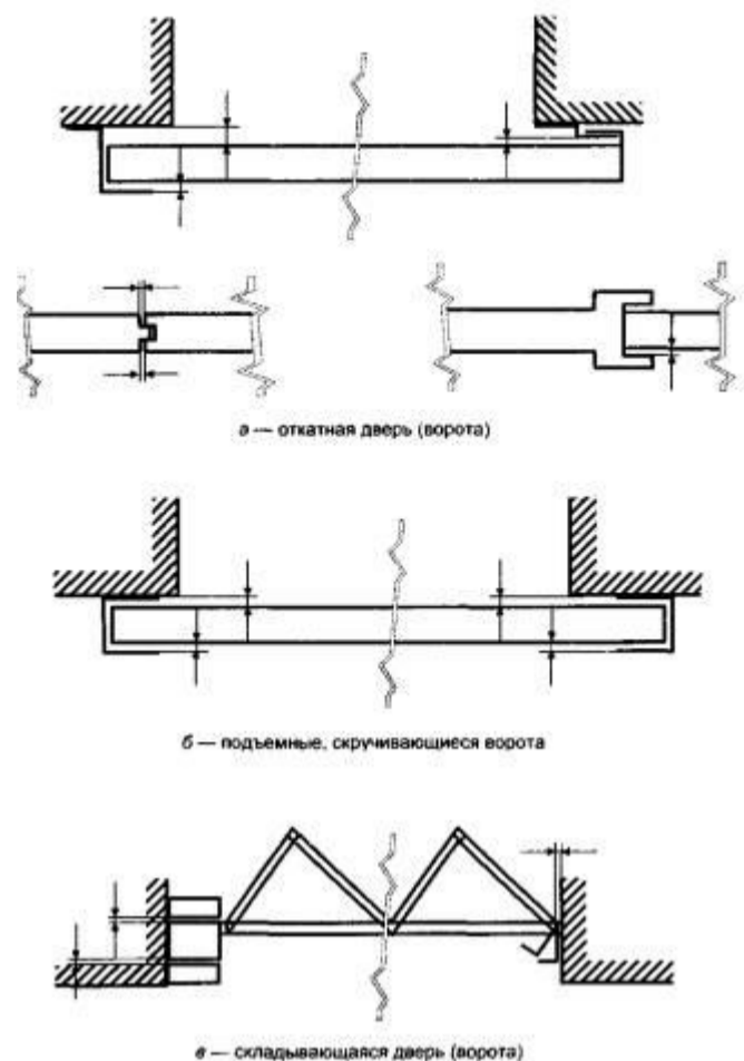
Рисунок 26 - Примеры замеров зазоров (горизонтальное сечение)
