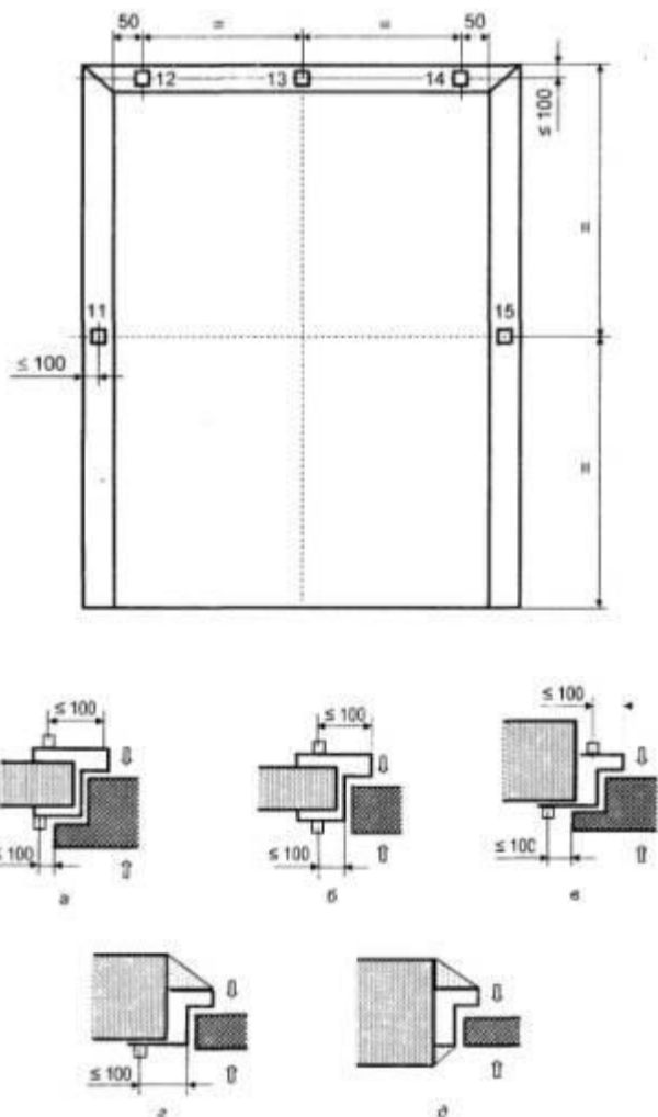
Рисунок 16 - Схема установки термодпар на необогреваемых поверхностях полотен подъемных и скручивающихся ворот
