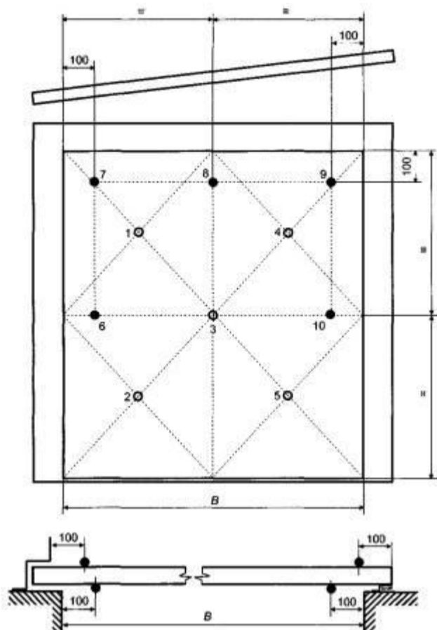
Рисунок 13 - Схема установки термодатчиков на необогреваемой поверхности полотна распашной двупольной двери в районе среднего притвора (горизонтальное сечение)
